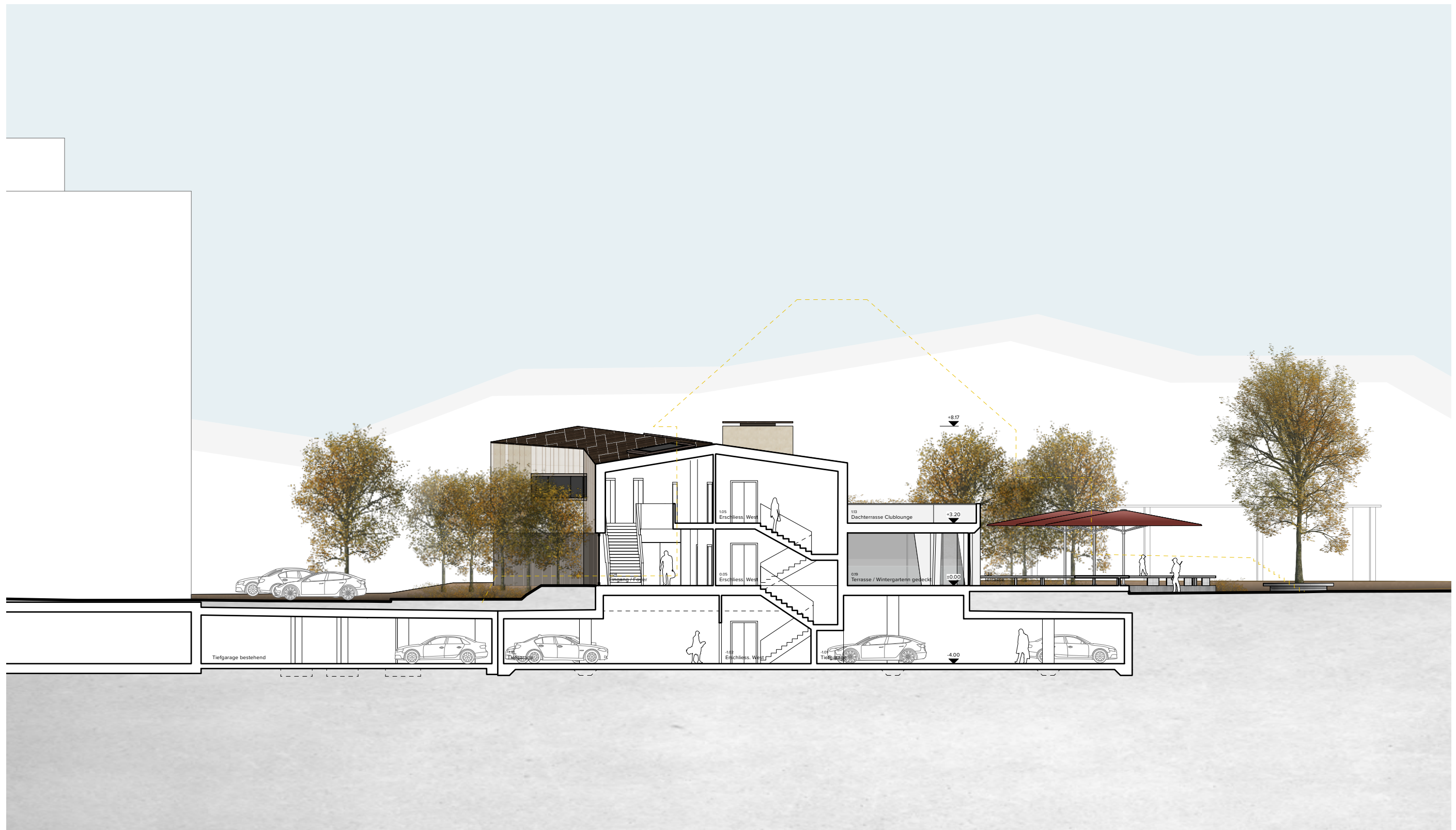
Querschnitt A-A
